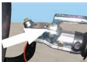
Bild: Verschleißanzeige Kugelkupplung
