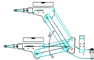
Bild: Höhenverstellbare Zugdeichsel
